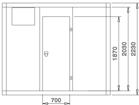
Zij aanzicht
